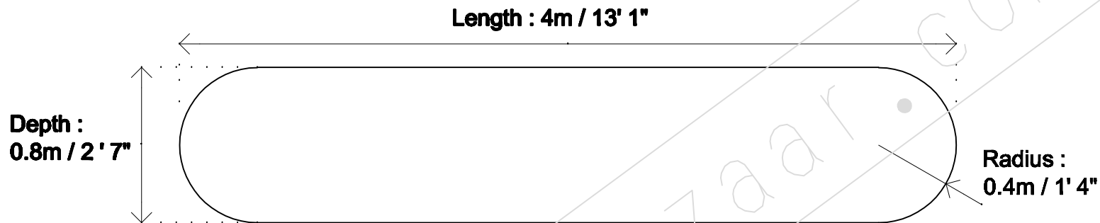
Ruber : plan
